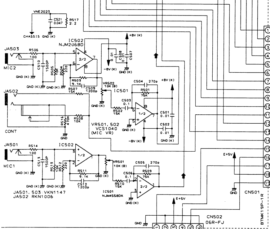
JACB ASSY VWV1422
