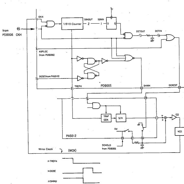
FIG. 15-5-6
