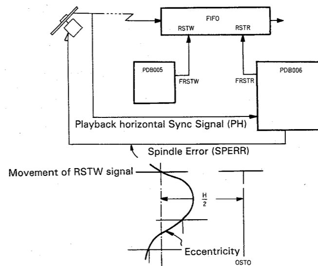
FIG. 15-5-13
